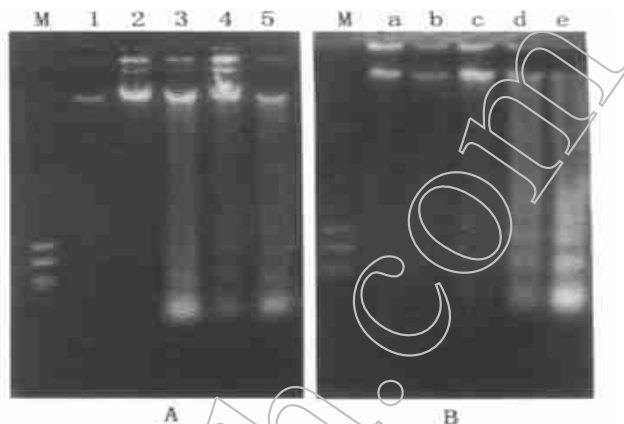
图 4 DNA 琼脂糖电泳结果
